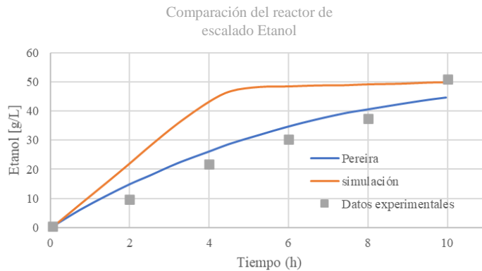
Figura 14. Comparación del escalado en la producción de etanol en el tiempo de Pereira et al, datos experimentales [8] y la realizada en este artículo.
