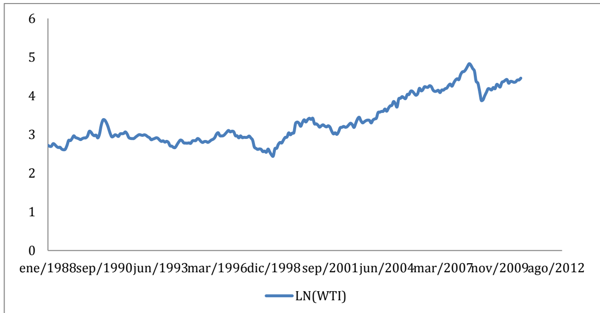
GRÁFICO 7: REGRESIÓN
